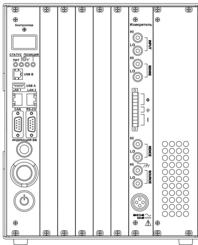
Рисунок 2а – Внешний вид изделия (вид спереди)
