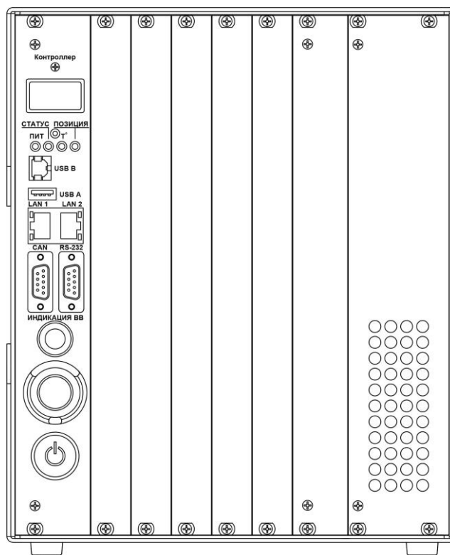
Рисунок 3а – Внешний вид изделия (вид спереди)
