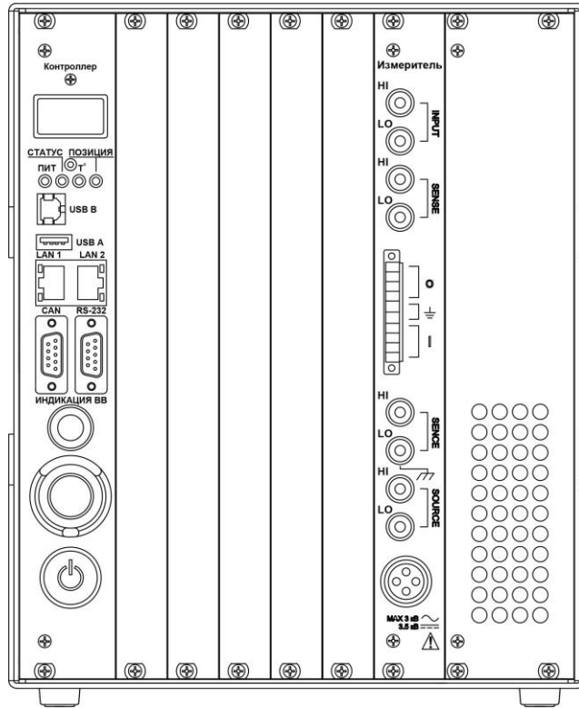
Рисунок 1а – Внешний вид изделия (вид спереди)
