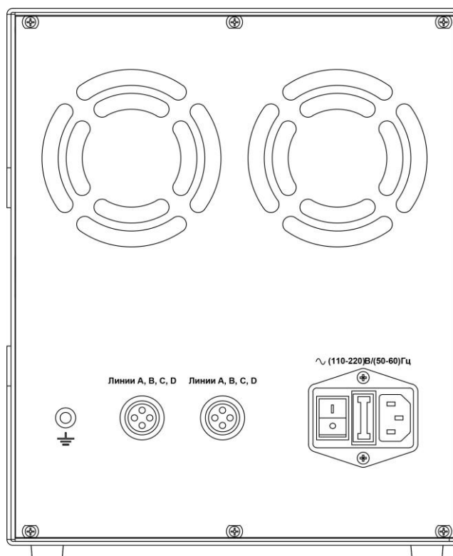
Рисунок 3б – Внешний вид изделия (вид сзади)
